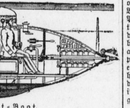
Das Holland-Boot.
