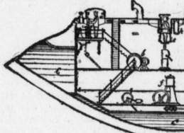
Fischtorpedo.
