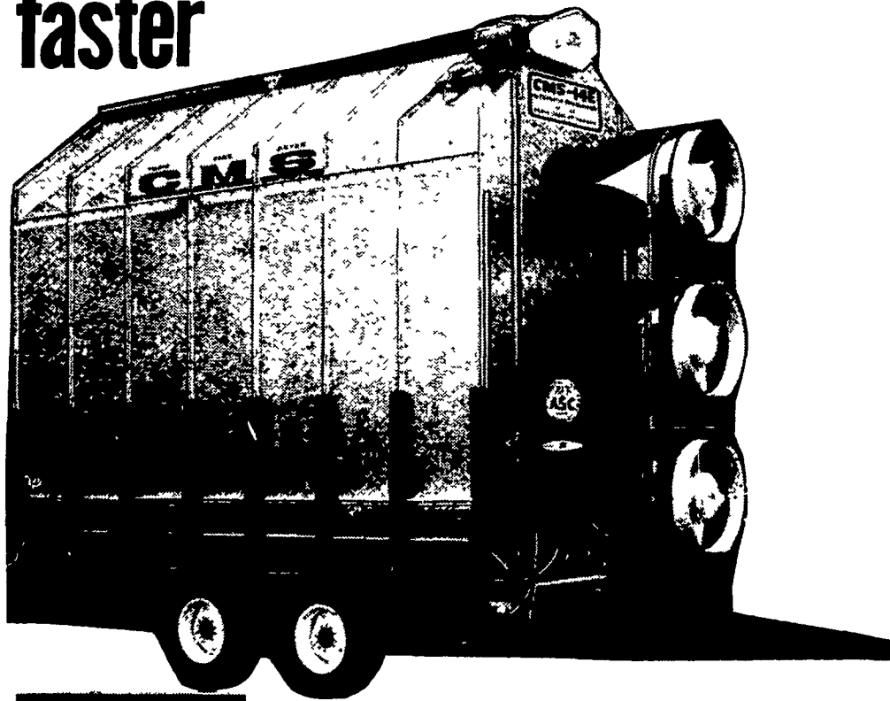
CMS Model—14E Temper Dries to 450 bu. per hr.
